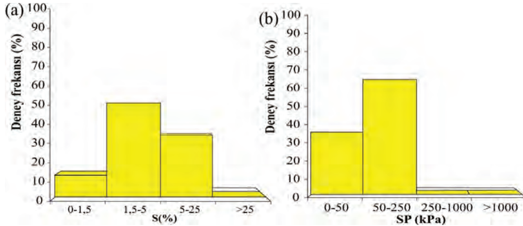
Şekil 11. Gündül zemin örneklerinin a) hacimsel değişim histogramı b) şişme basıncı (kPa) histogramı (Wayne vd., 1994).
